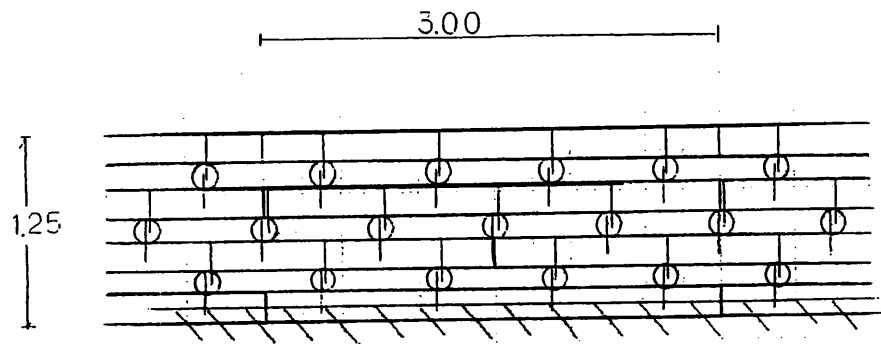
3段組土羽止丸太組工
