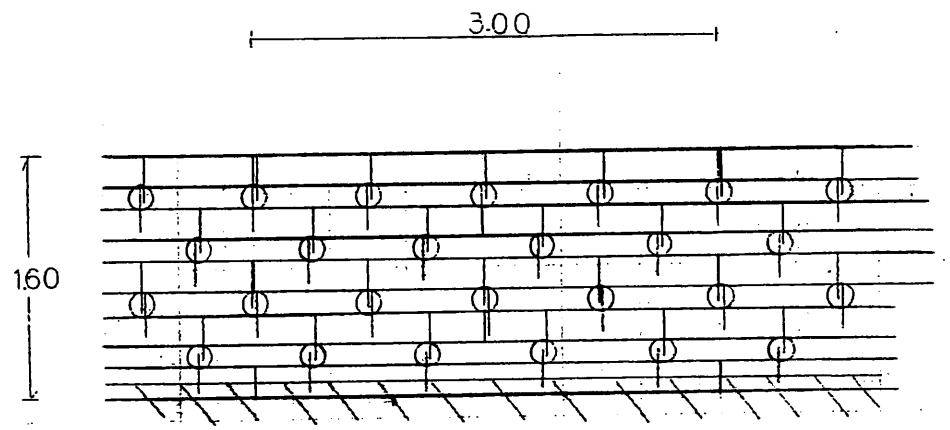
4段組土羽止丸太組工
