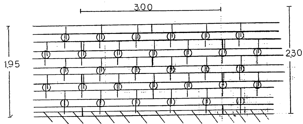
5段組土羽止丸太組工
